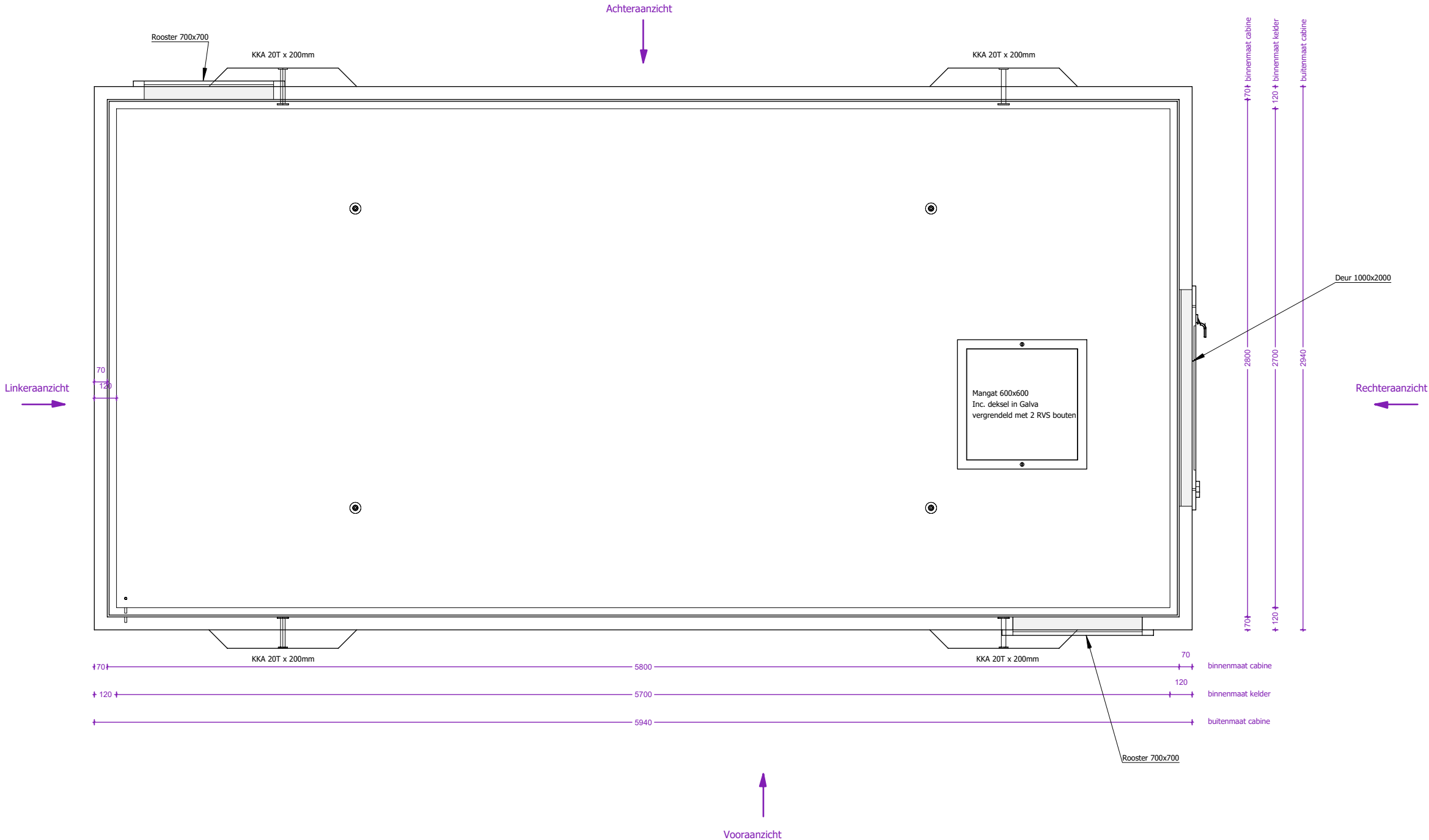
Bovenaanzicht
