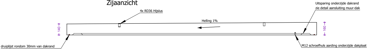
Zijaanzicht
