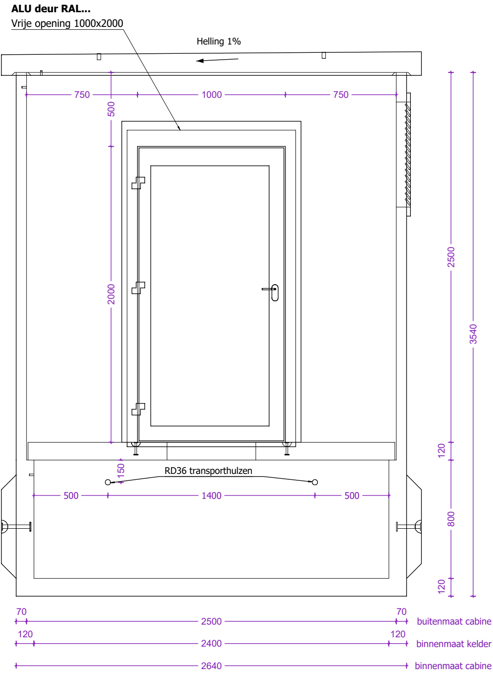
Linkerzijaanzicht
