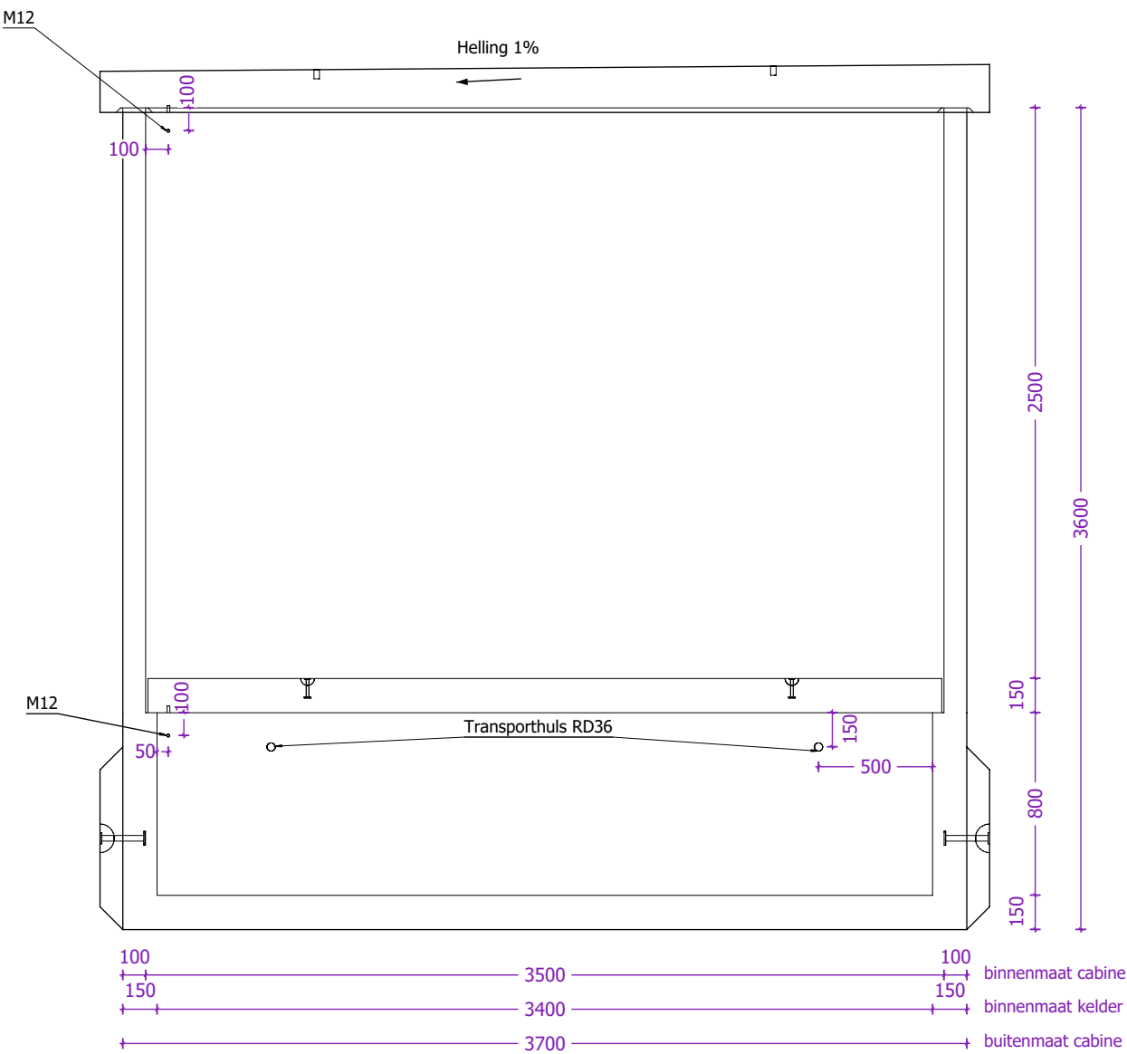
Rechterzijaanzicht
