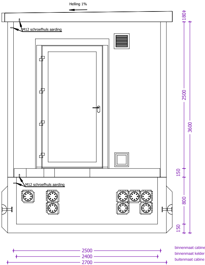
Vooraanzicht
