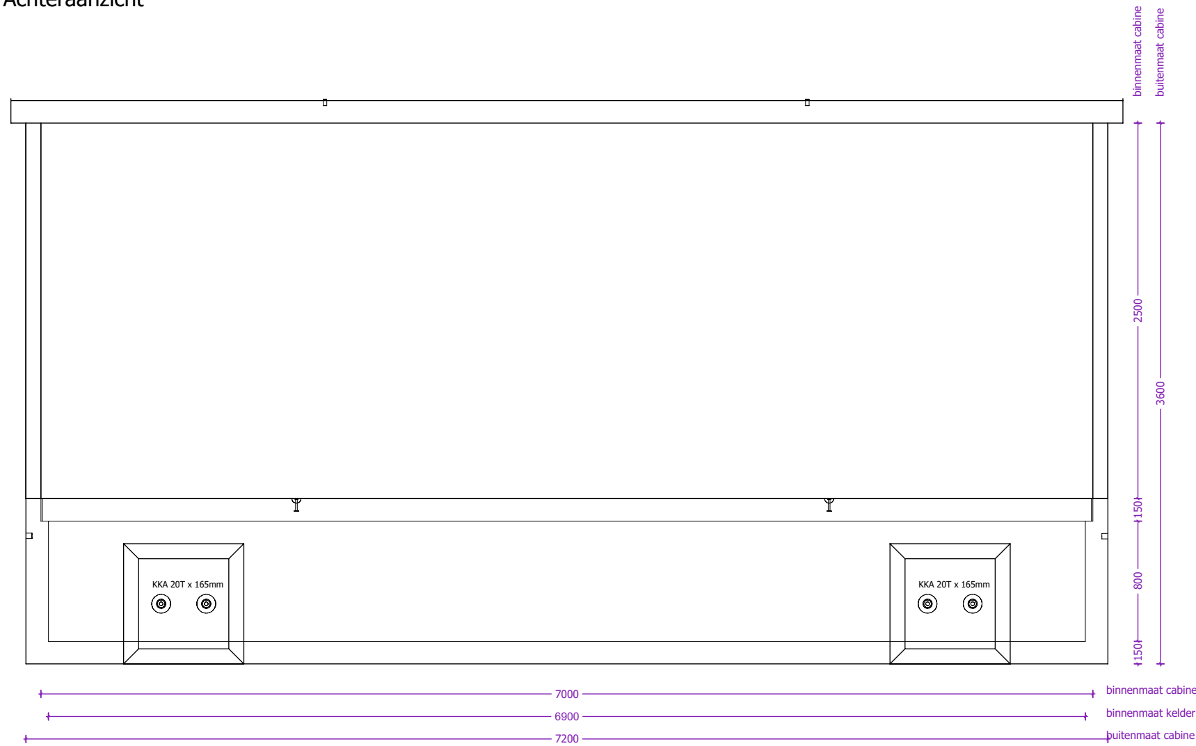
Achteraanzicht
