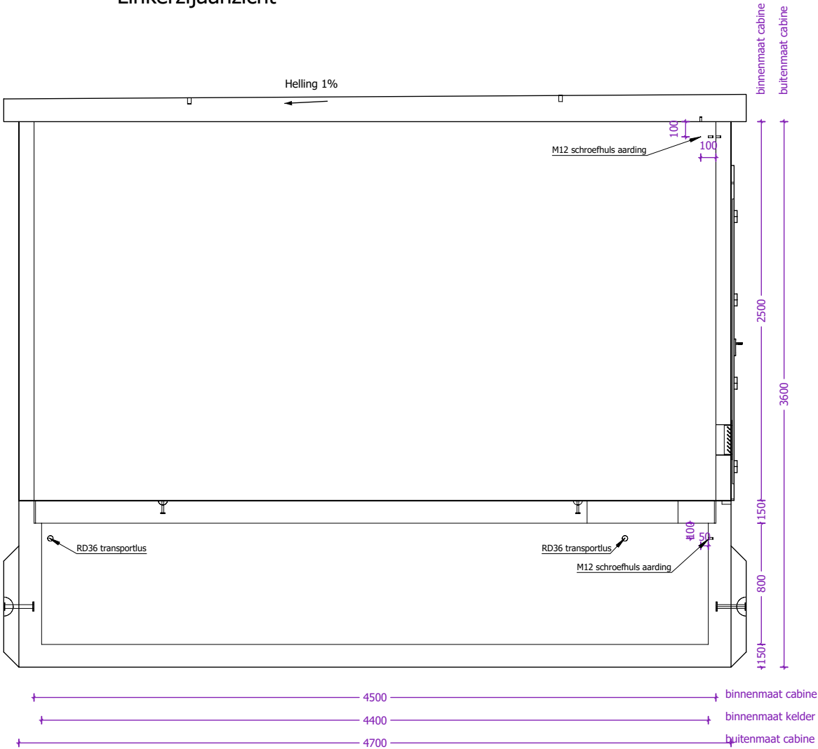
Linkerzijaanzicht
