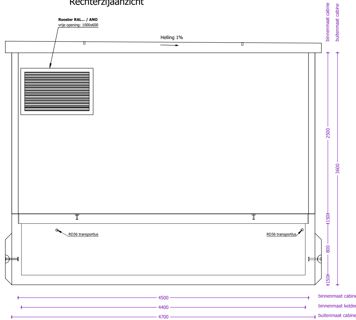
Rechterzijaanzicht
