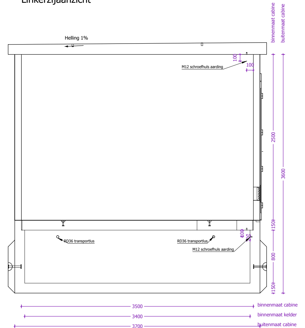
Linkerzijaanzicht
