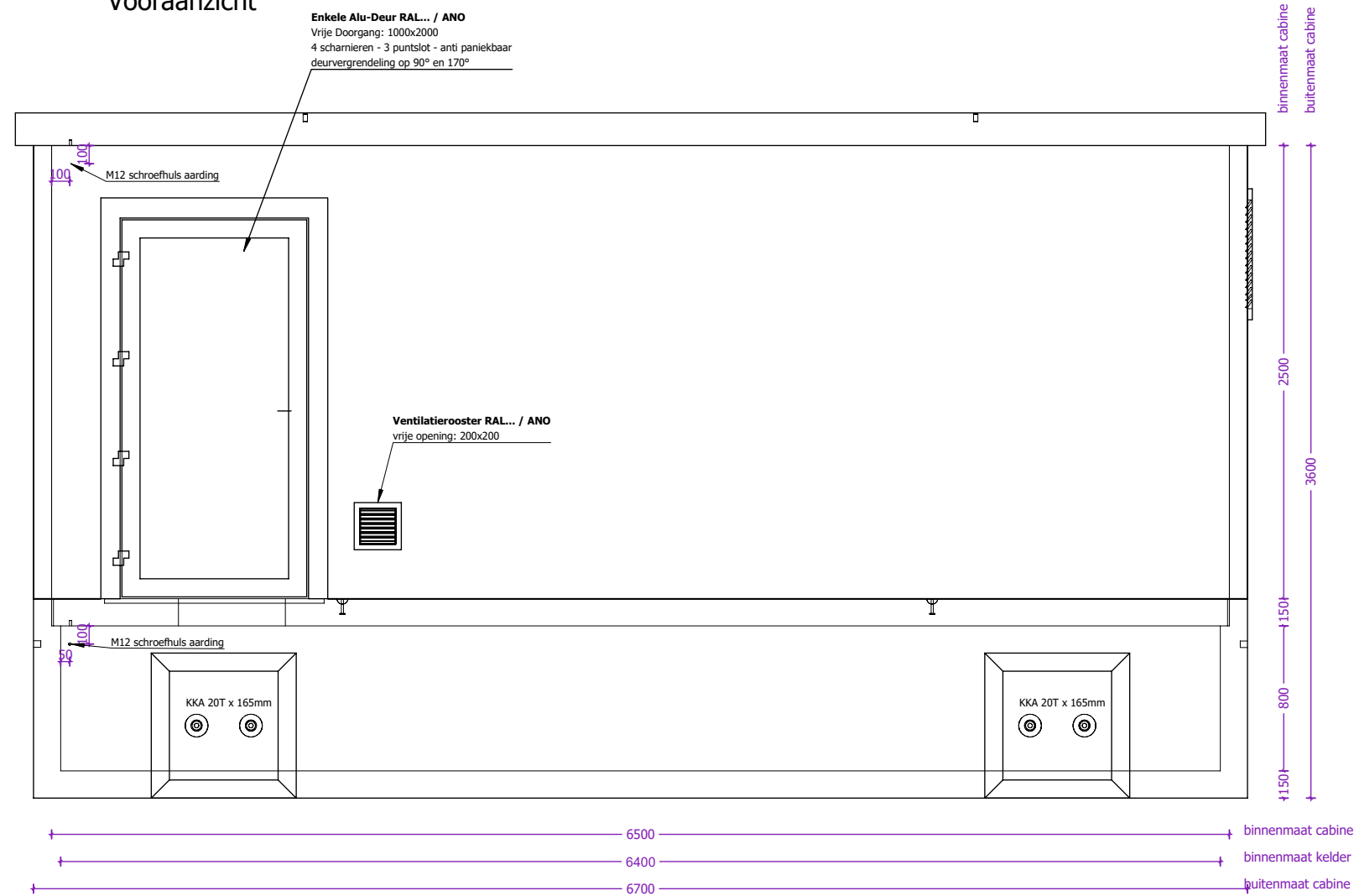
Vooraanzicht
