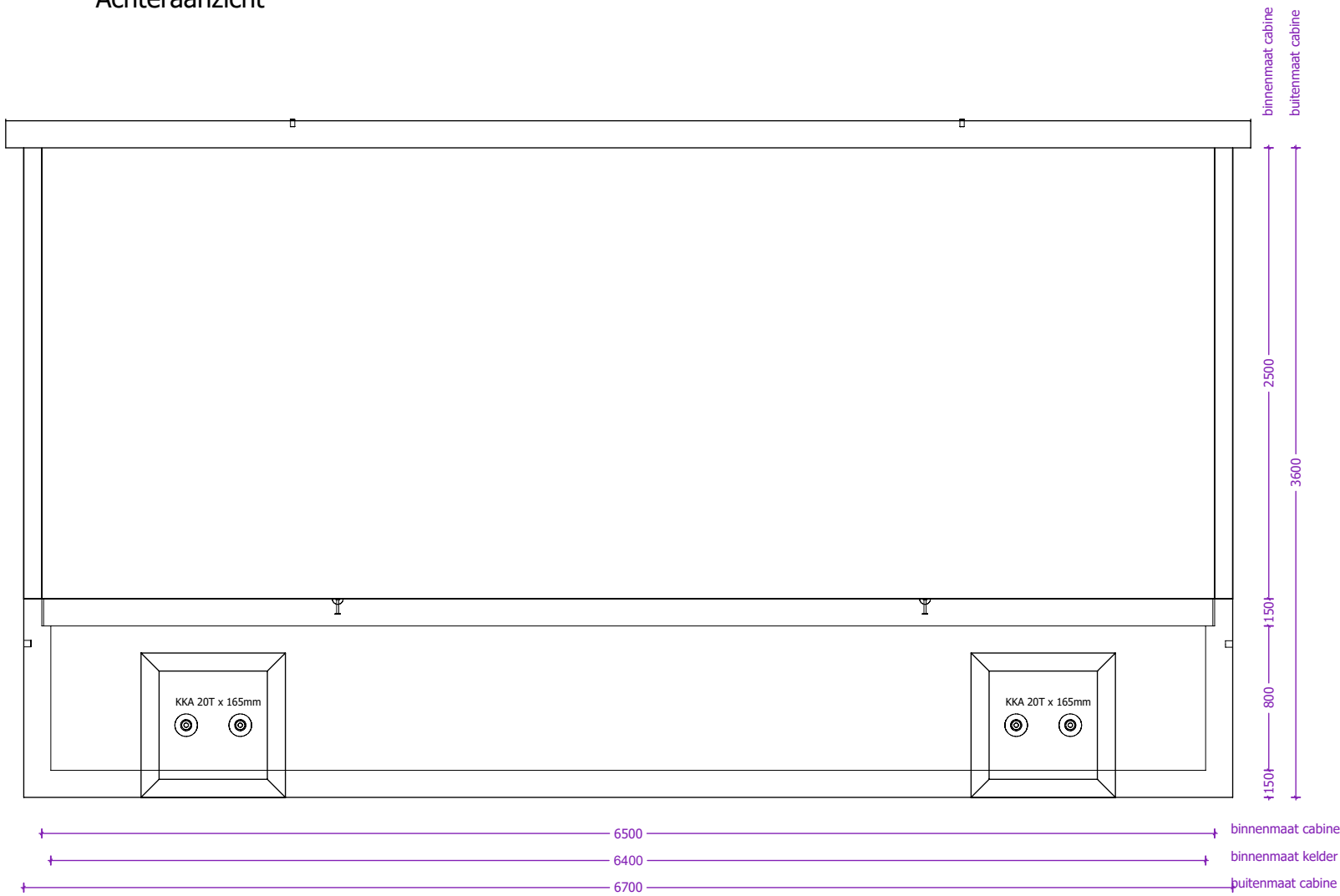
Achteraanzicht
