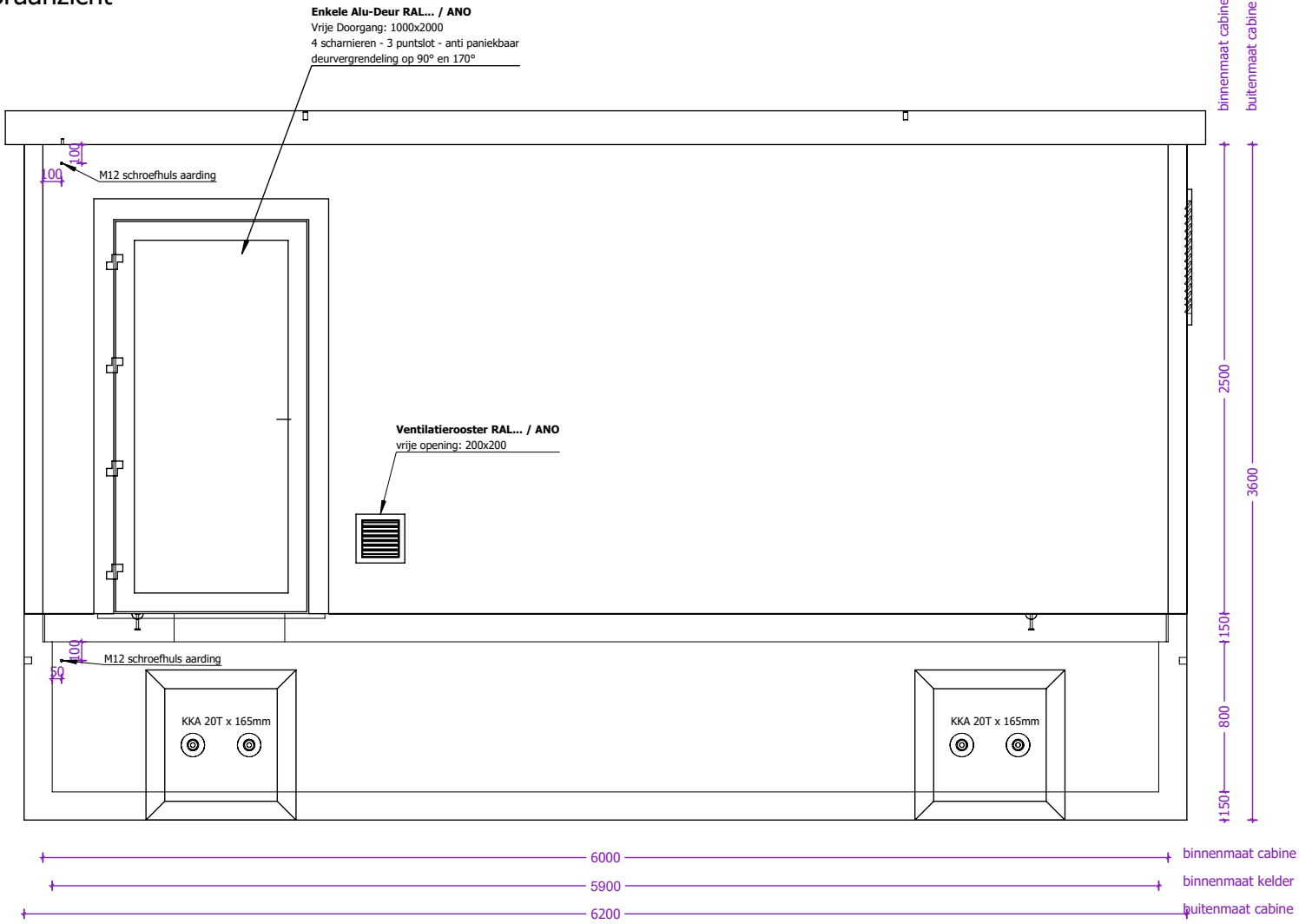
Vooraanzicht
