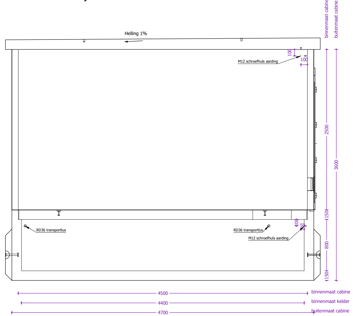
Linkerzijaanzicht
