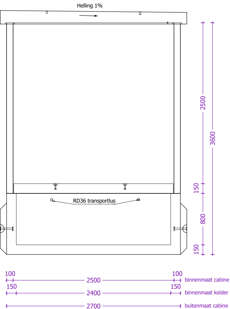
Rechterzijaanzicht
