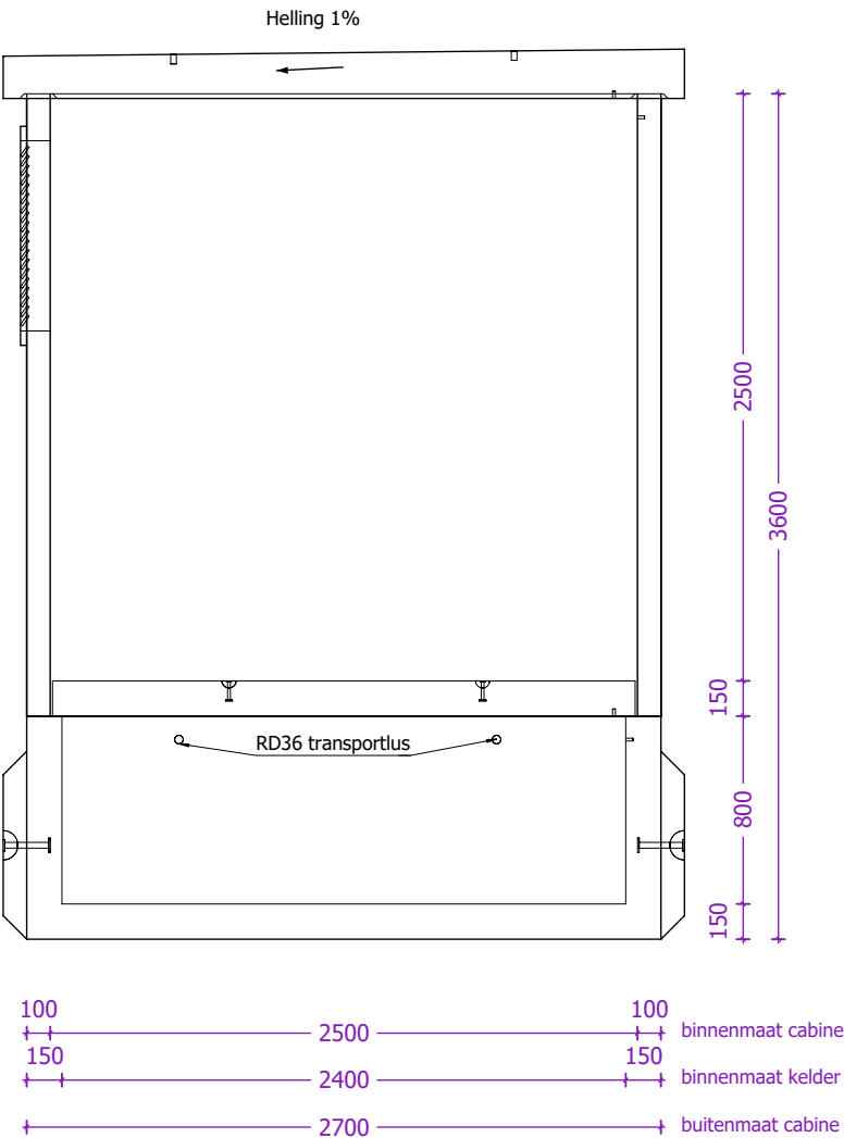
Linkerzijaanzicht
