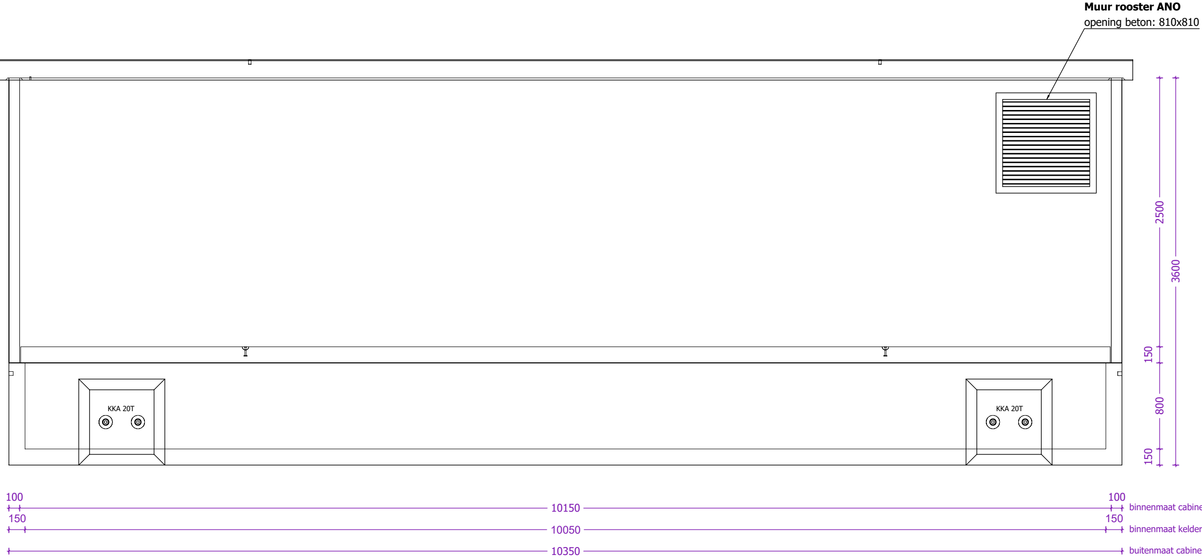
Achteraanzicht
