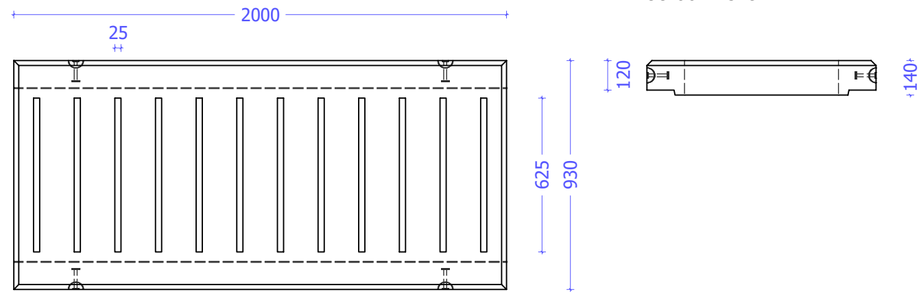
Vooraanzicht
