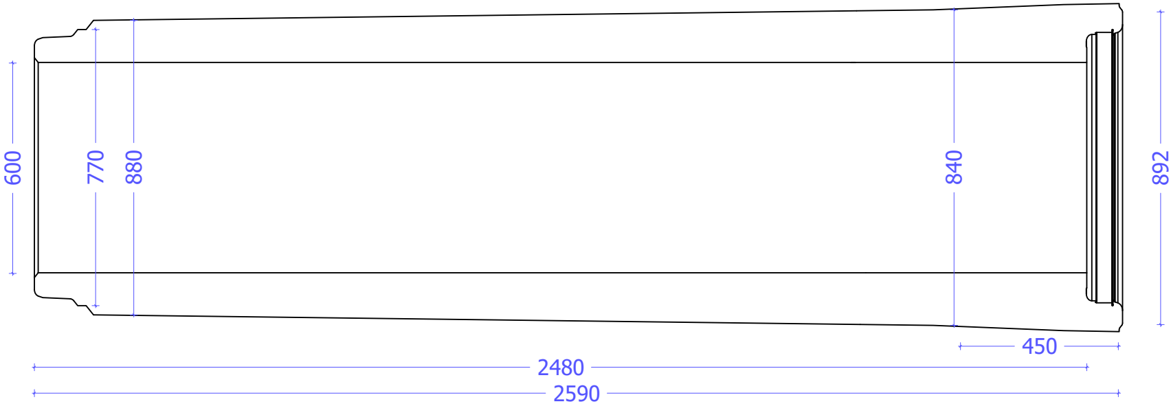
Standaard buis
