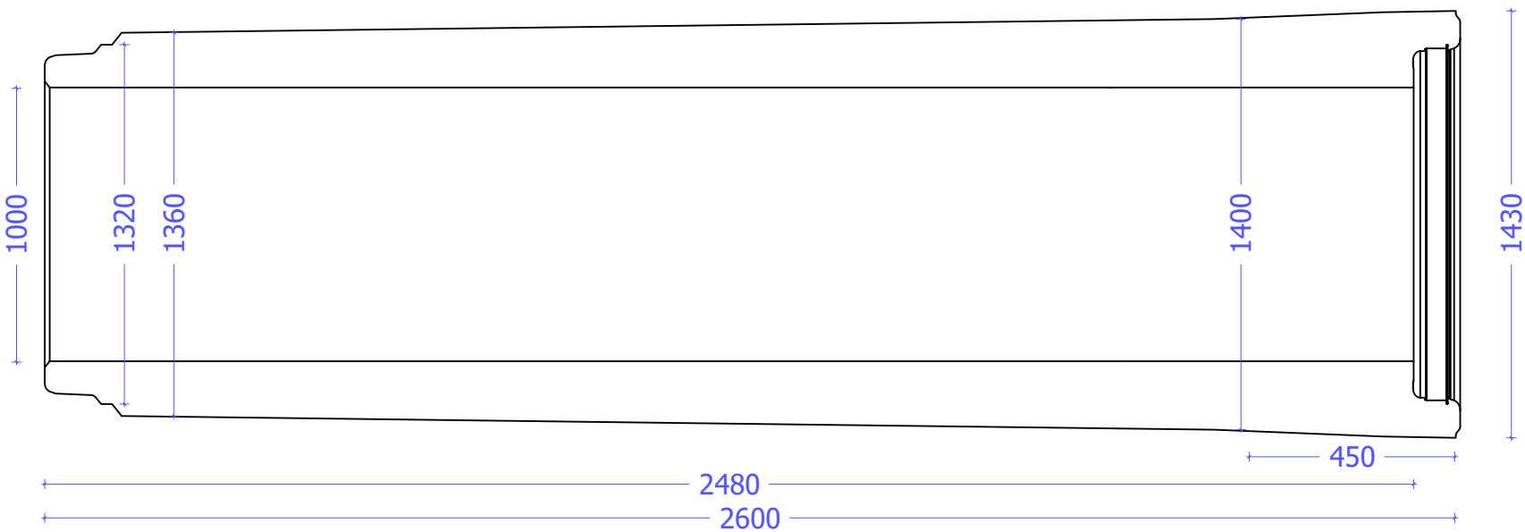
Standaard buis
