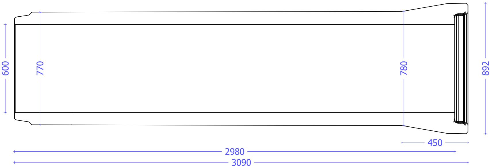
Standaard buis
