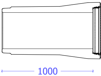
Ongewapende pendelbuis
