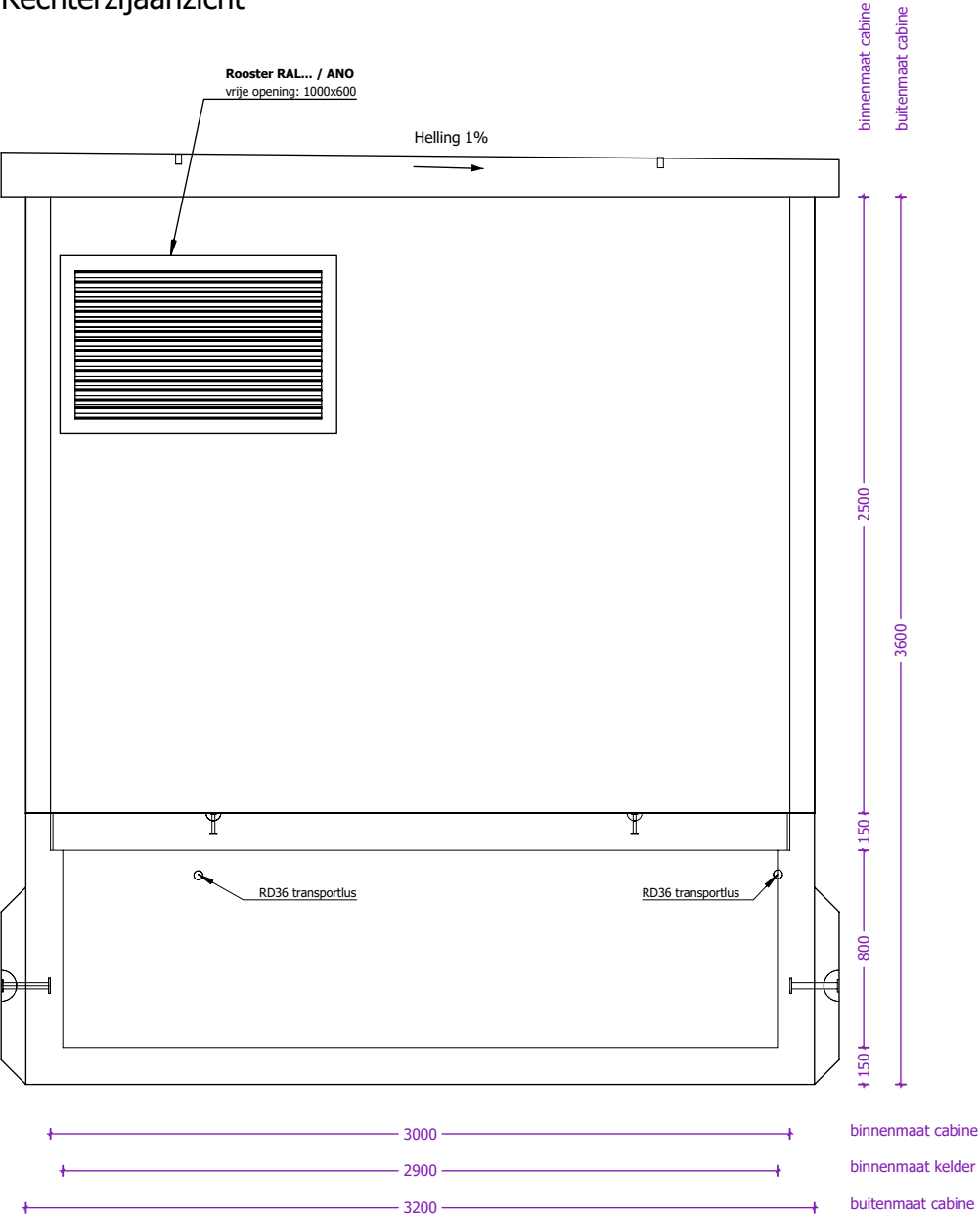
Rechterzijaanzicht
