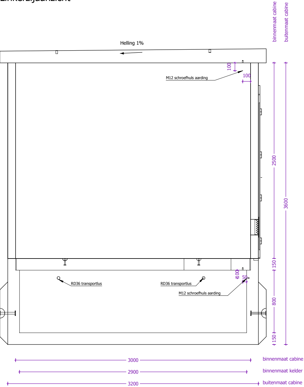
Linkerzijaanzicht
