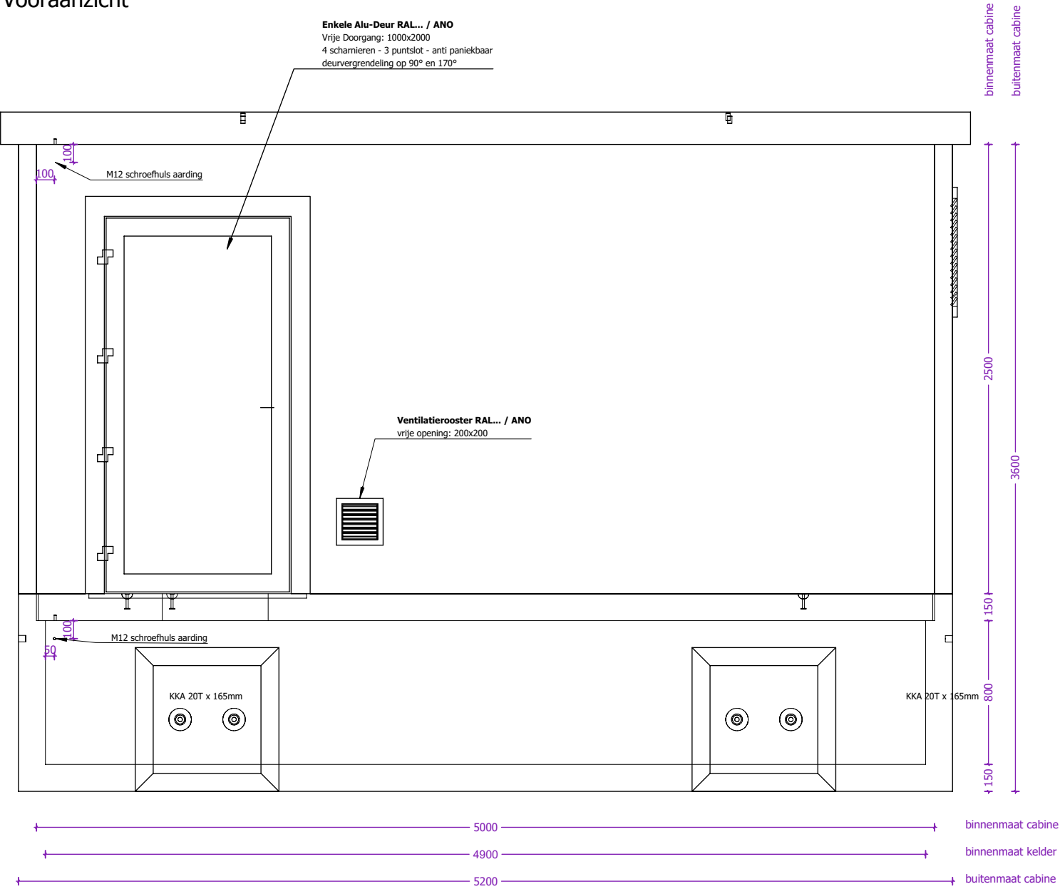
Vooraanzicht
