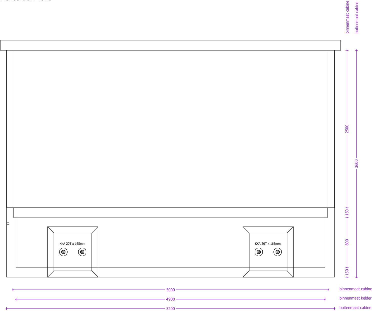
Achteraanzicht
