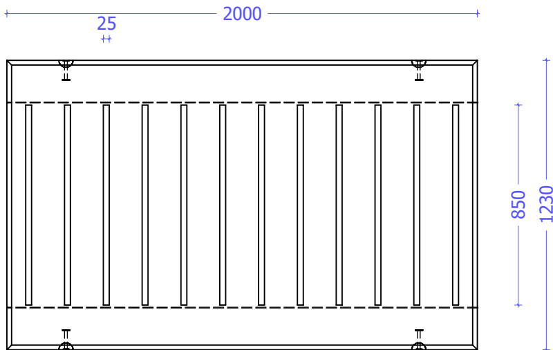
Bovenaanzicht
