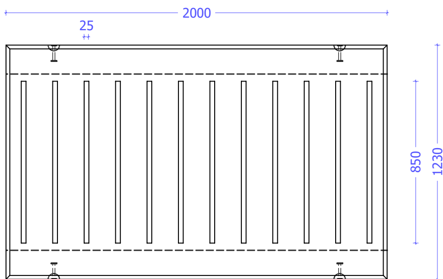
Bovenaanzicht
