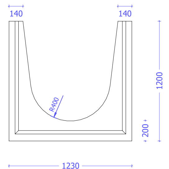
Vooraanzicht
