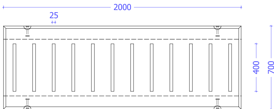
Bovenaanzicht
