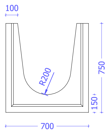
Vooraanzicht
