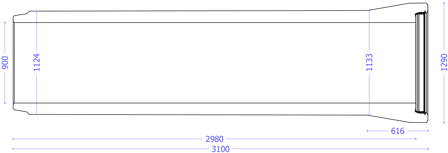
Standaard buis
