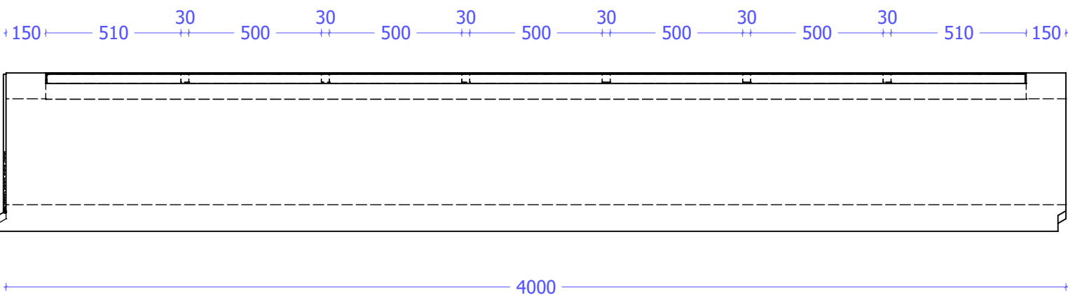
Zijaanzicht
