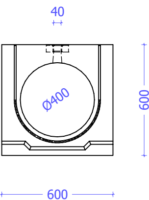
Vooraanzicht
