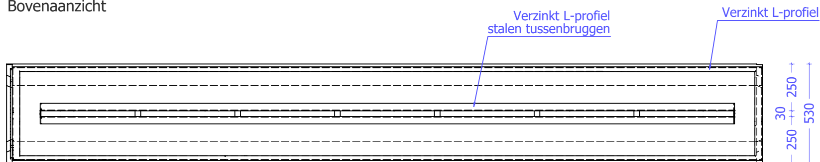
Bovenaanzicht
