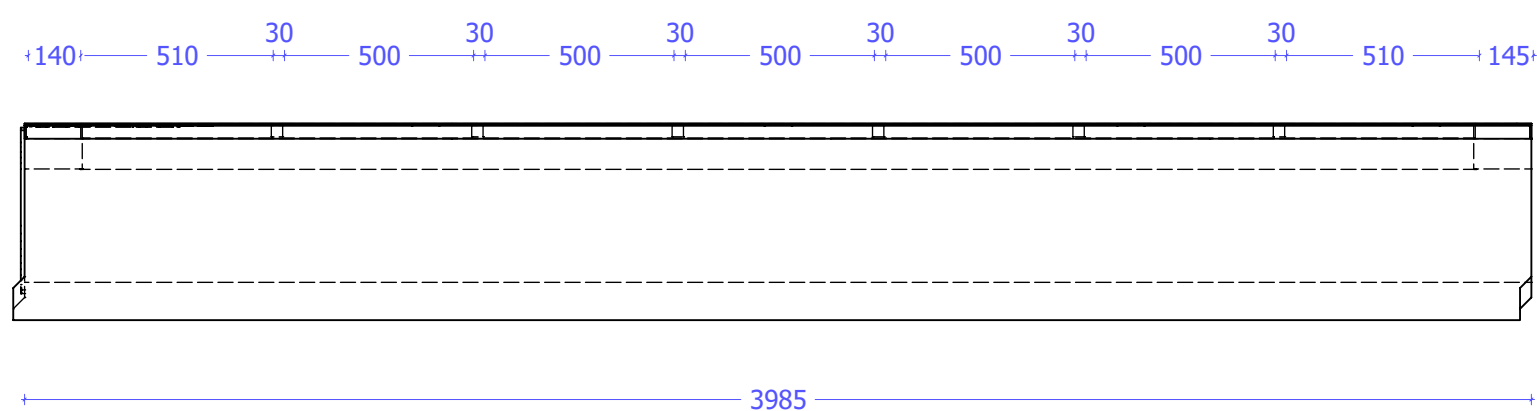
Zijaanzicht
