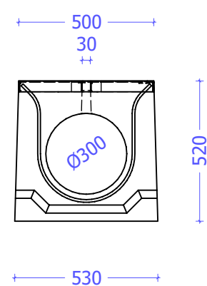
Vooraanzicht
