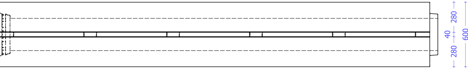
Bovenaanzicht
