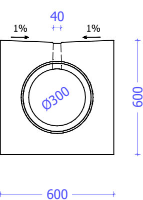
Vooraanzicht
