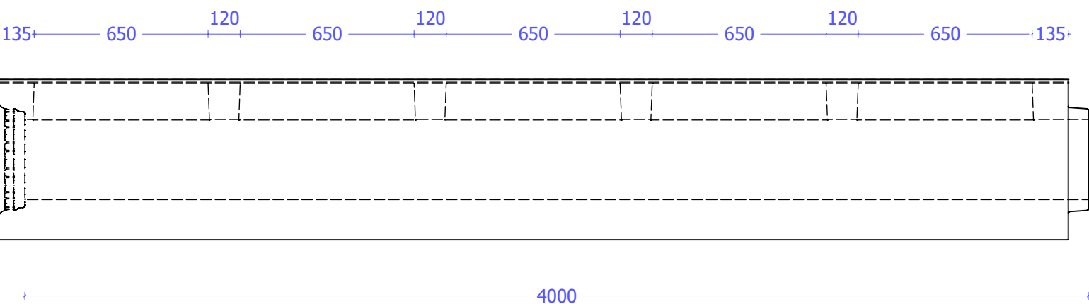
Zijaanzicht
