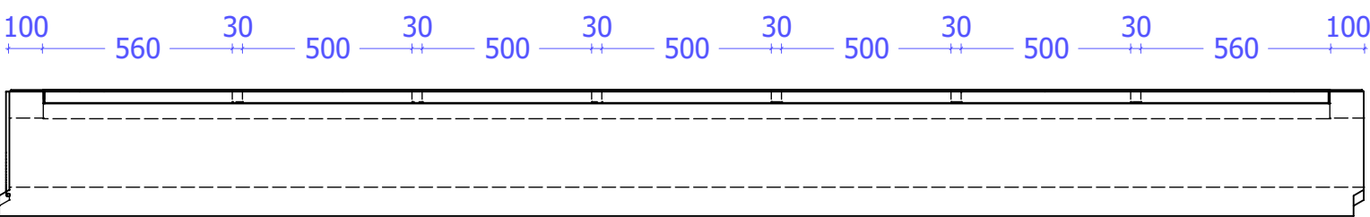
Zijaanzicht
