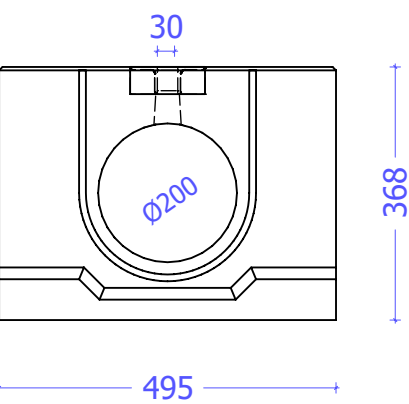
Vooraanzicht
