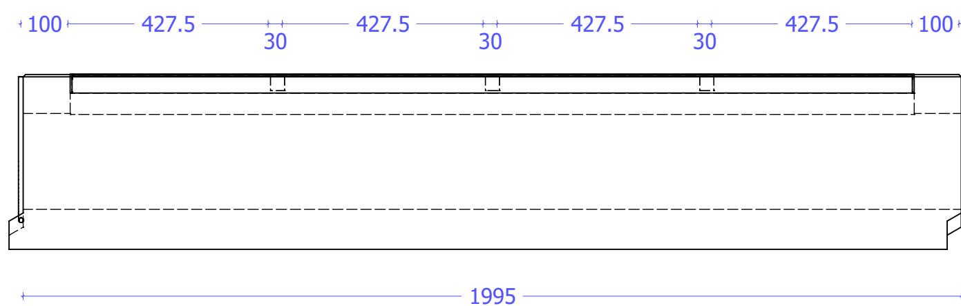
Zijaanzicht
