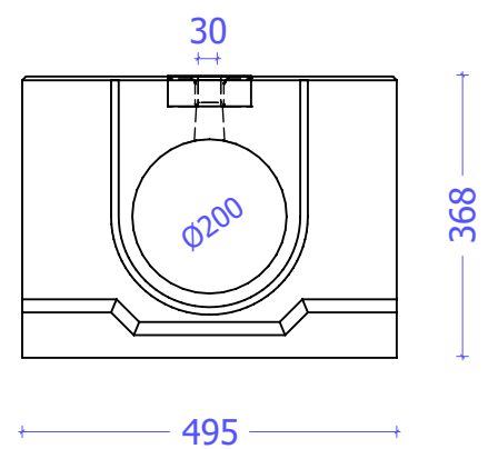
Vooraanzicht
