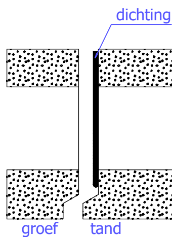
Bovenaanzicht
