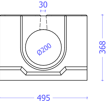
Vooraanzicht
