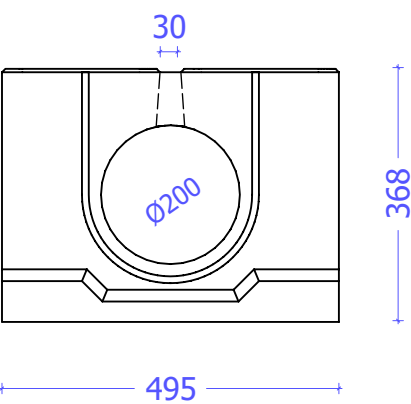
Vooraanzicht
