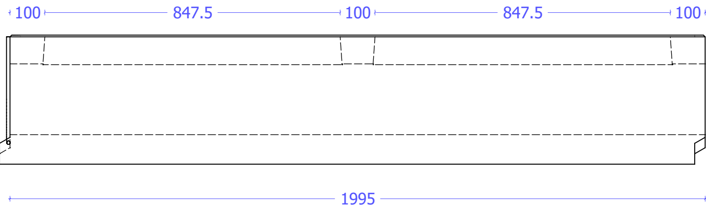
Zijaanzicht
