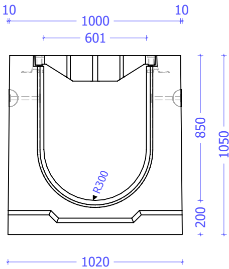
Vooraanzicht
