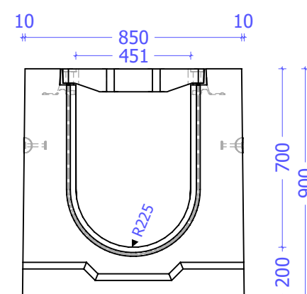
Vooraanzicht
