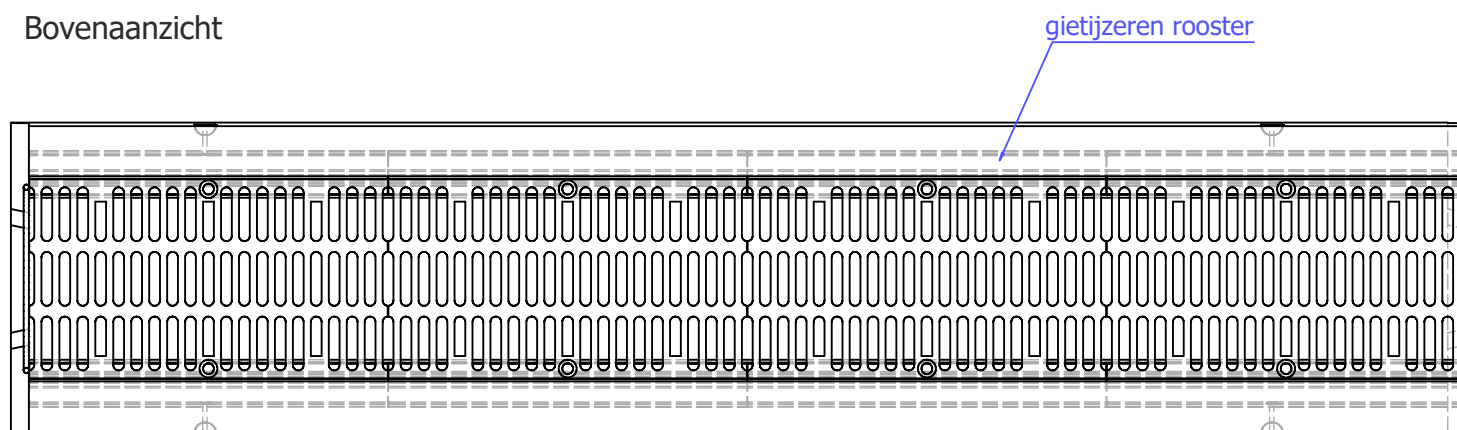
Zijaanzicht
