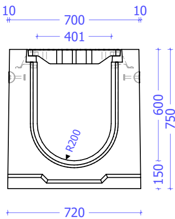
Vooraanzicht
