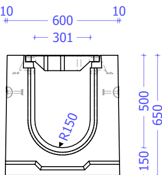
Vooraanzicht
