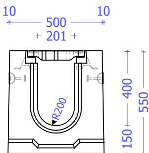
Vooraanzicht
